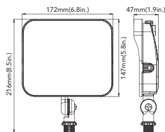
15W&27W(Knuckle Mount)
